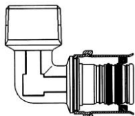
Press külső menetes könyök
